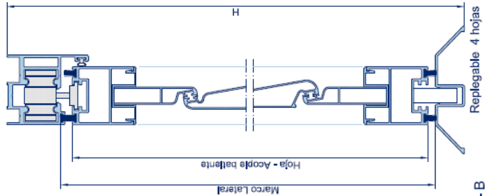
SECCION B - B
