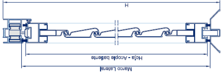
SECCION B - B
